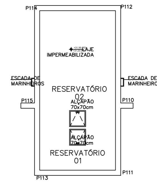
PLANTA BAIXA CX. D'AGUA ESCALA 1:100
