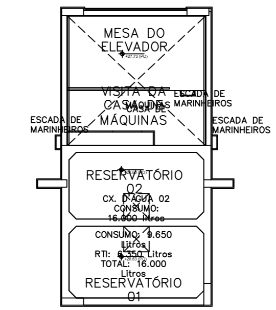
PLANTA BAIXA RESERVATORIO ESCALA 1:100
