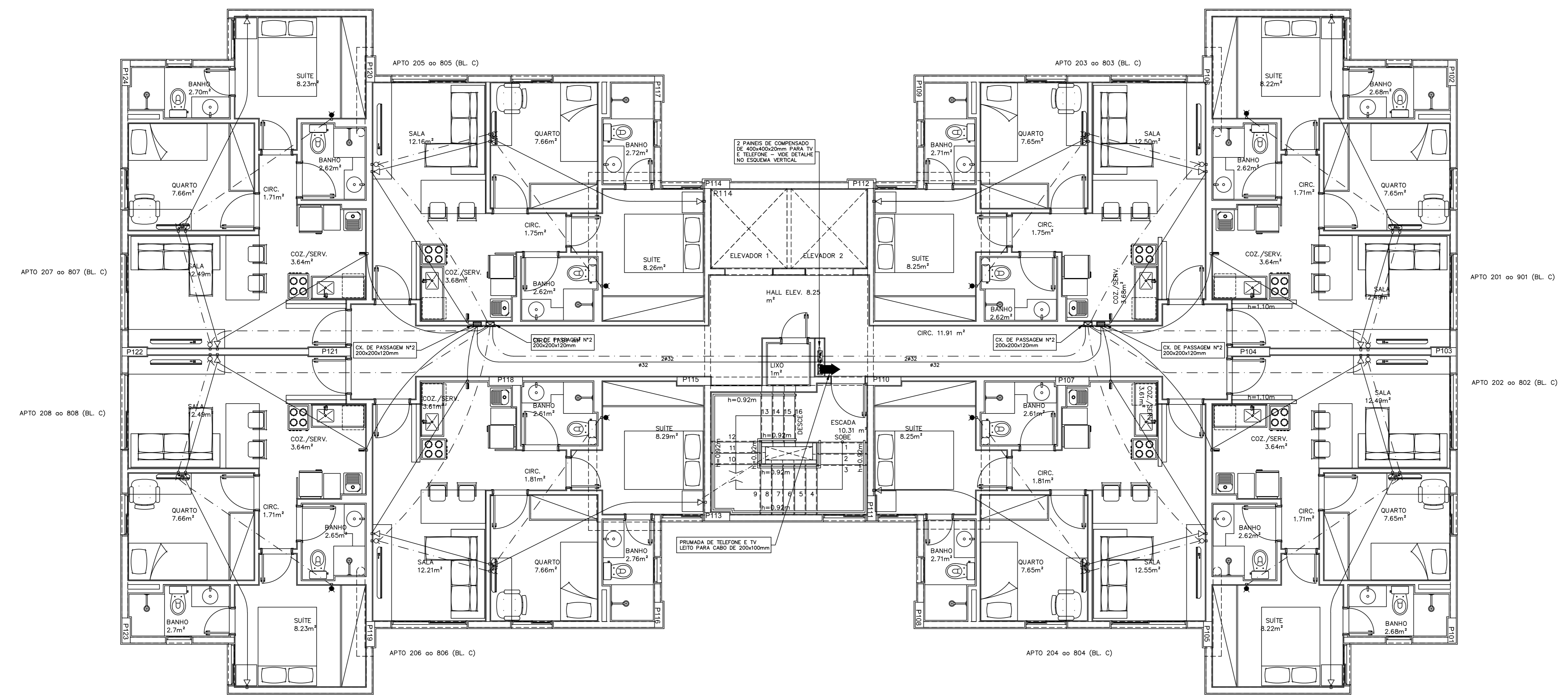
PLANTA BAIXA PAVIMENTO TIPO BLOCO C ESCALA 1:50
